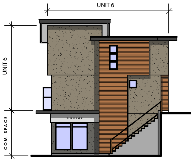
RIGHT ELEVATION
